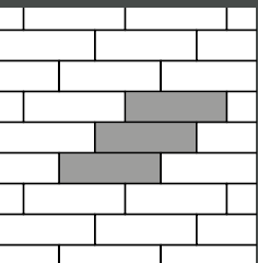
Drittelverband
