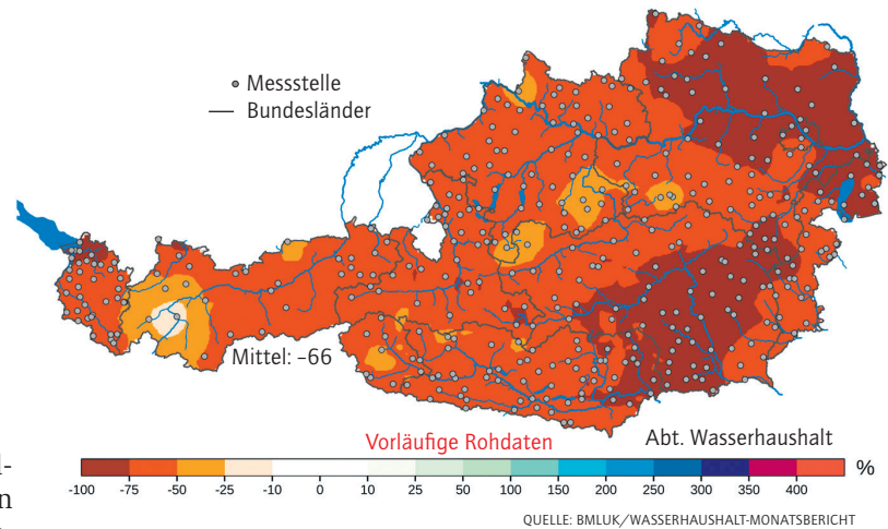
Abweichung des Monatsniederschlags im April 2026 vom langjährigen Monatsmittel (1991-2020)
