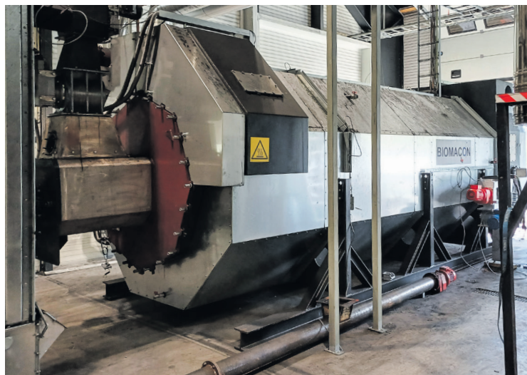
Herzstück der Produktion ist der Bioreaktor. Dort erfolgt die Pyrolyse.
