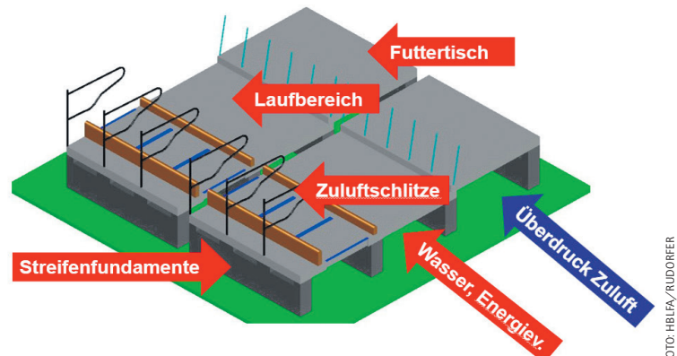
Unterflurzuluft ist eine Lösung zur Kühlung des Liegebereiches.
