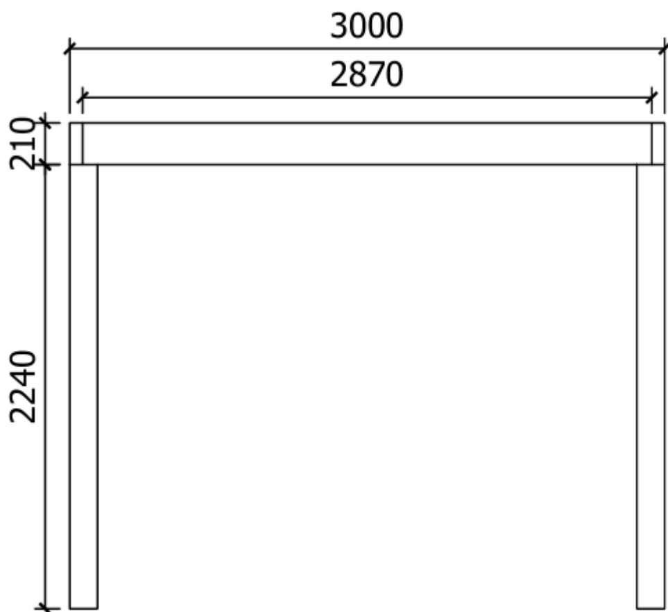
Zijaanzicht
