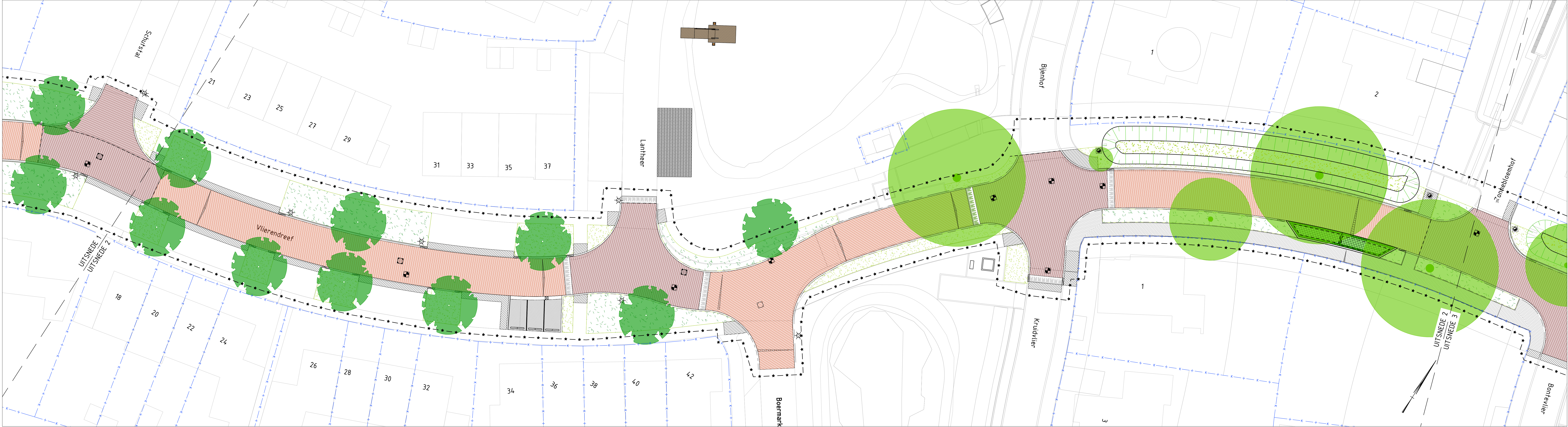
UITSNEDE 2 SCHAAL 1 : 200
