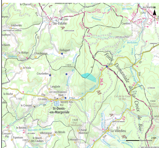
Localisation des points de mesure acoustique autour du projet éolien du Bois d'Apcher
