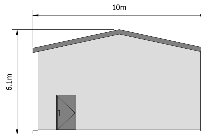
END ELEVATION
