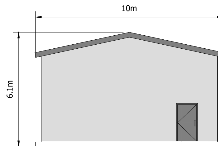
END ELEVATION
