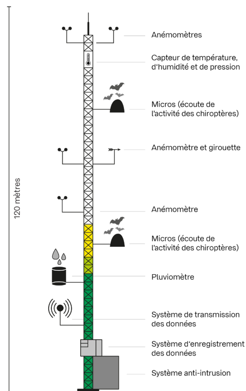
Schéma d'un mât de mesure
