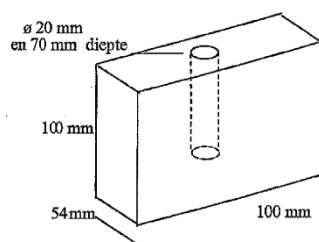
Fig. 1 – afmetingen van de proefstukken en uitvoering van het boorgat
