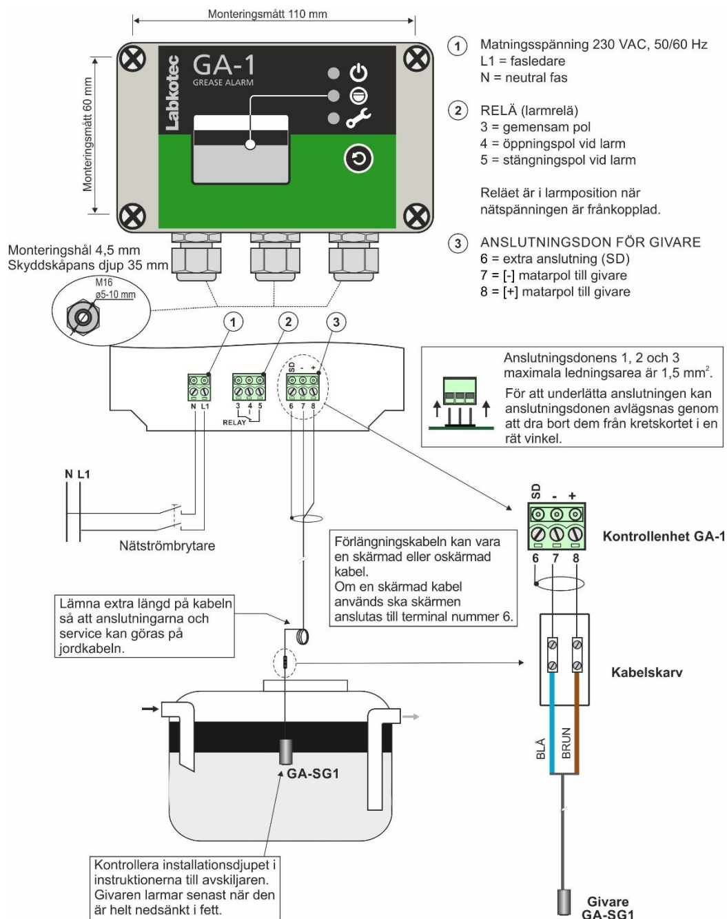
Bild 3. Installation av larmanordning GA-1.
