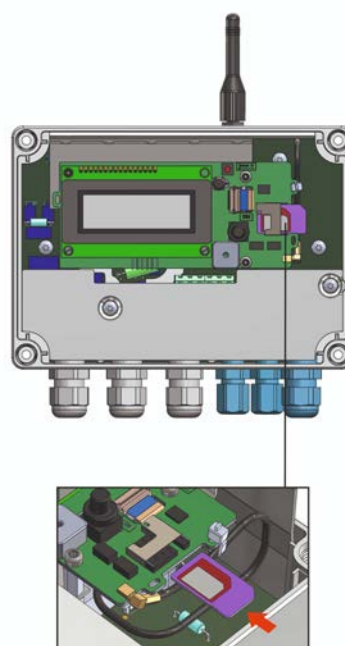
Bild 22. Installation av SIM-kort
