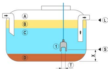
Bild 12. Installera idOil-SLU-slamgivaren
