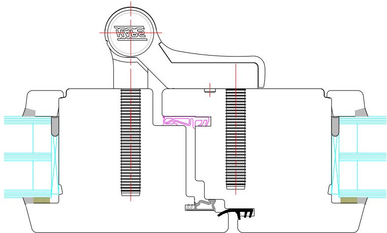
Hinge Jamb
