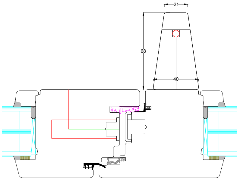
Handle Jamb
