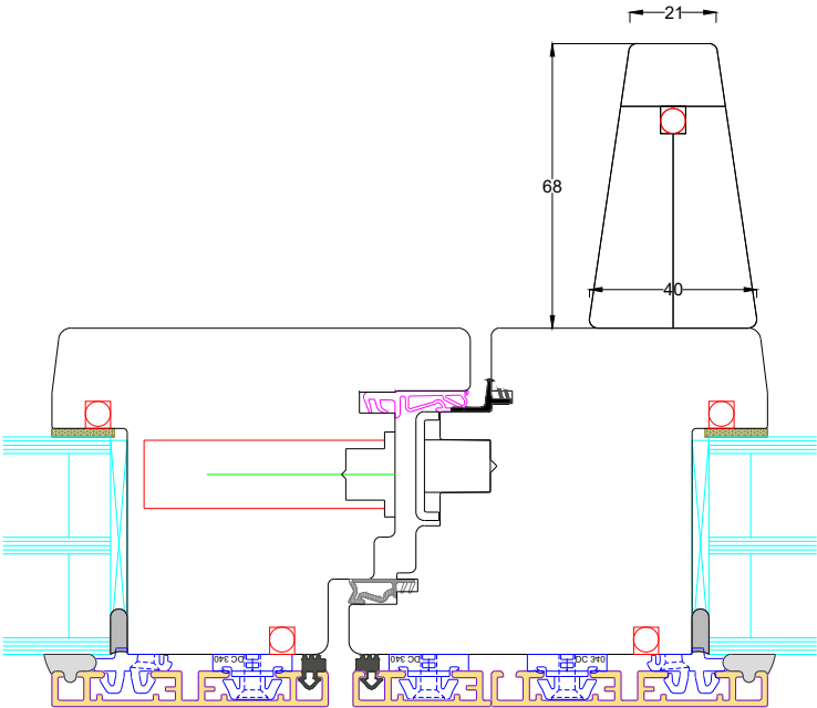
Handle Jamb
