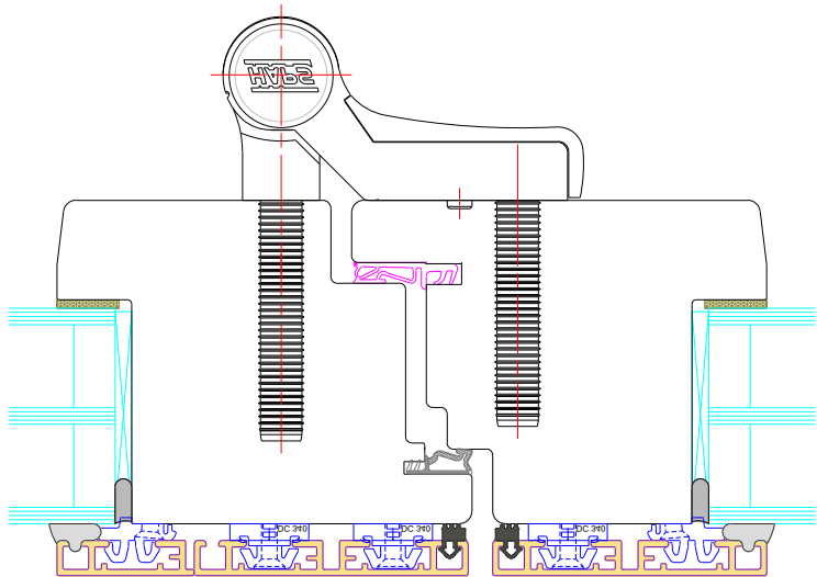
Hinge Jamb
