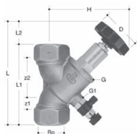
1530 Schrägsitzventil mit Entleerung und Handrad, PN16, für Wasser bis 90°C Nyffenegger Robinet oblique à vidage et volant, PN16, pour eau jusqu'à 90°C
