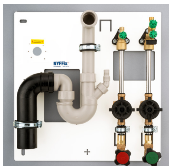
7900 G/D – Avec compteurs d'eau et robinets d'arrêt – Dimension 1/2" femelle NPK / Suissetec 222.817
