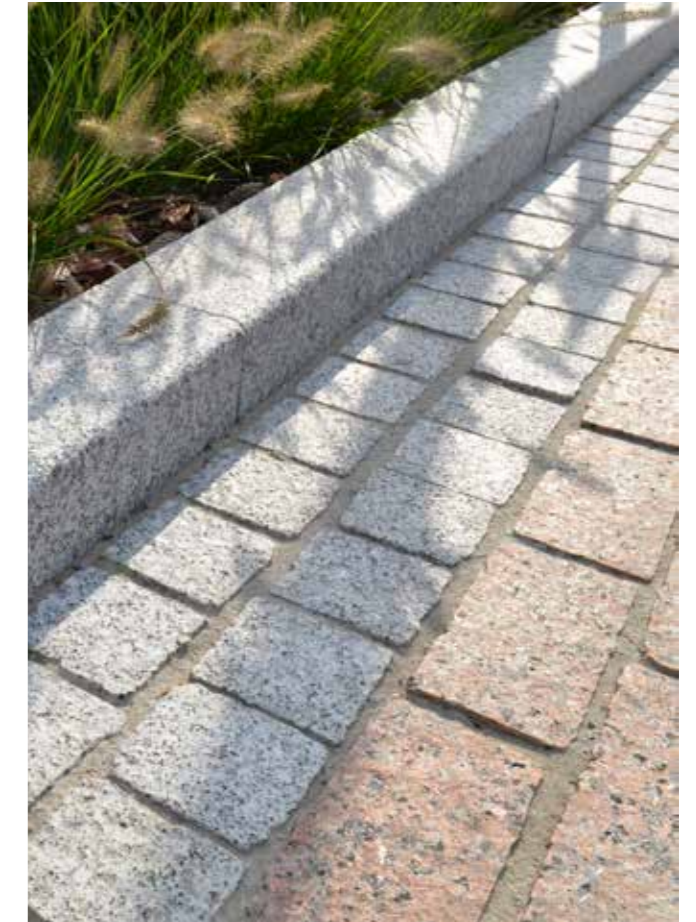
boordsteen en plavuis links: Tarn - gevlamd plavuis rechts: Rose de la Clarté - gevlamd
