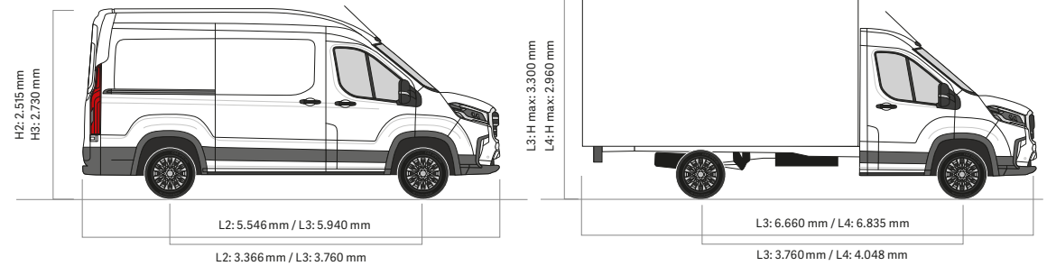
Maximale Abmessungen Fahrgestell inkl. Aufbau
