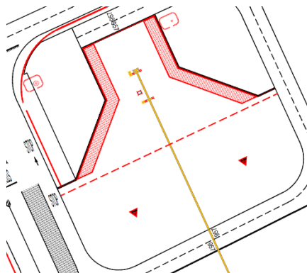
Fig. 9. Markering afbakening jet blast gevoelige zone
