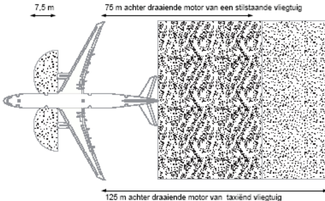
Fig. 33. Veiligheidsafstanden tot vliegtuigen met draaiende straalmotoren
