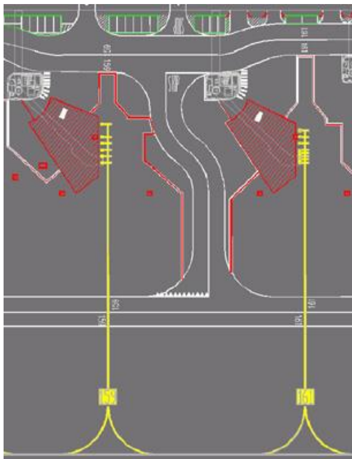
Fig. 11. Markeringen op de apron (159-161) Pier A met service drive voor- en achter vliegtuigstands
