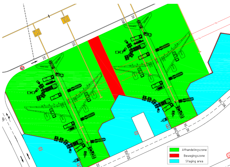
Fig. 32. Rode zone voorbij wingtips
