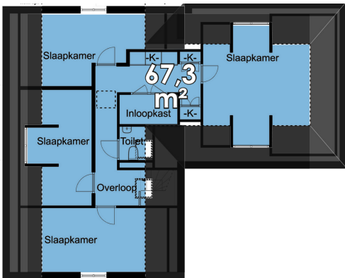
1e Verdieping
