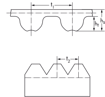
optibelt OMEGA RB im Querschnitt
