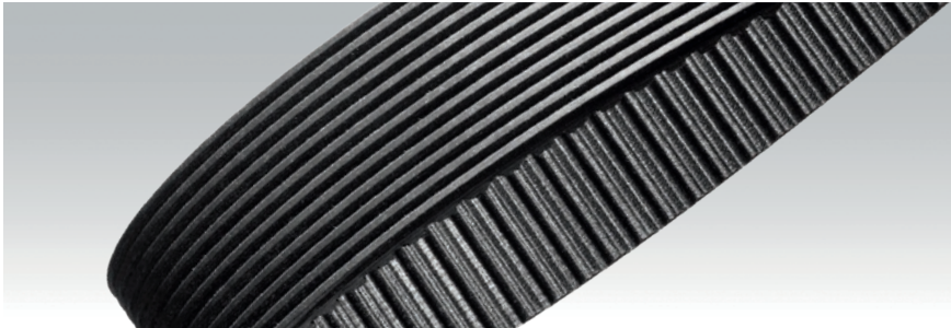
optibelt OMEGA RB im Querschnitt
