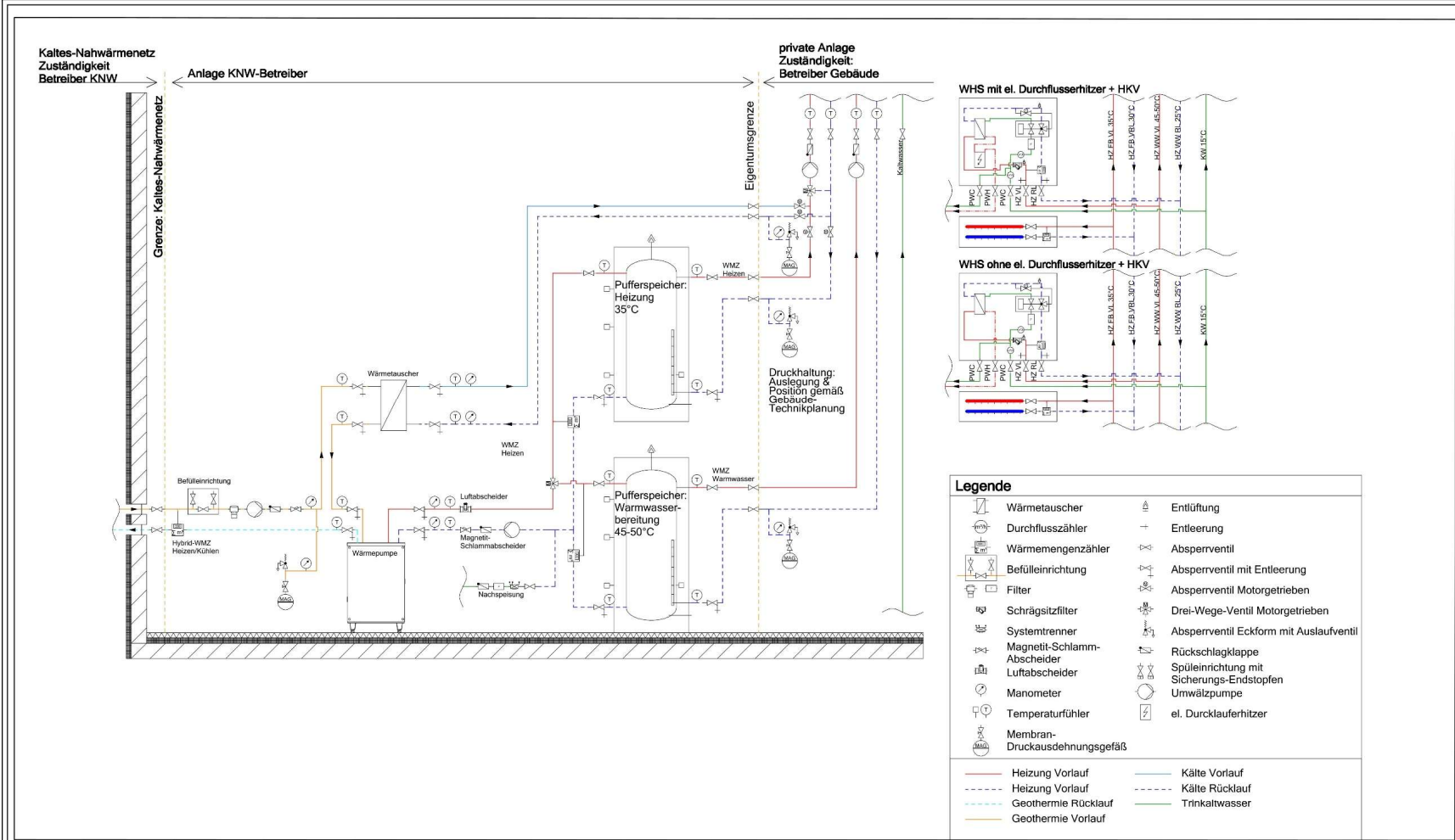
Schema Anschlussnehmer KNWN / MFH / hoher WW-Bedarf / Heizen + Freies Kühlen
