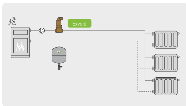
Sistema Ottone Exvoid – Schemi
