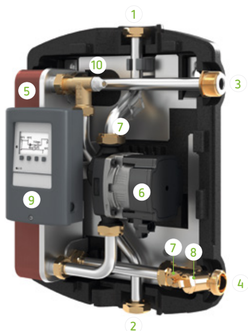
Reflex Hydroflow S – M modelli di produttori istantanei di ACS
