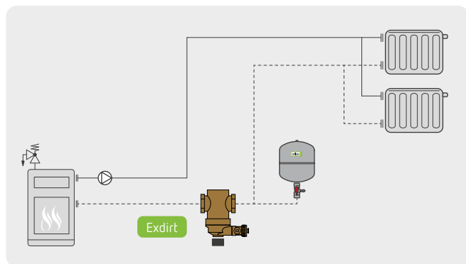
Sistema ottone Exdirt – Schemi
