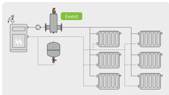
Sistema acciaio Exvoid – Schemi
