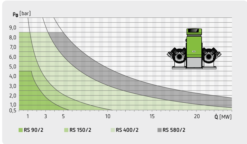
Reflexomat con due compressori
