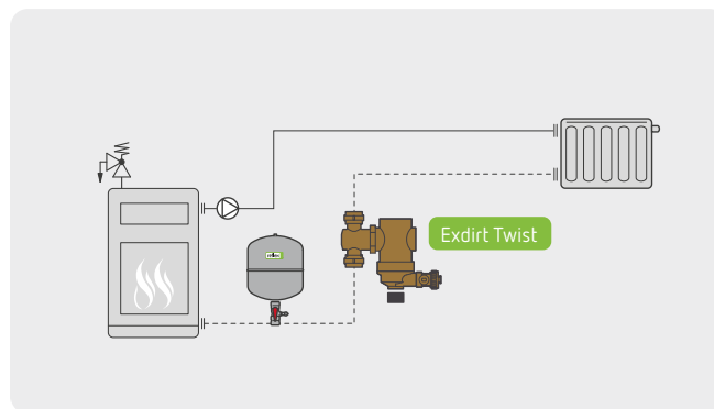
Sistema ottone Exdirt Twist – Schemi
