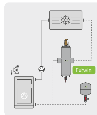
Sistema acciaio Extwin R – Schemi
