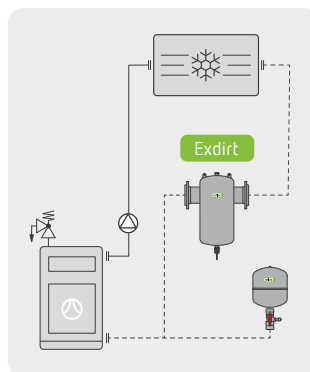
Système Exdirt acier – Schéma
