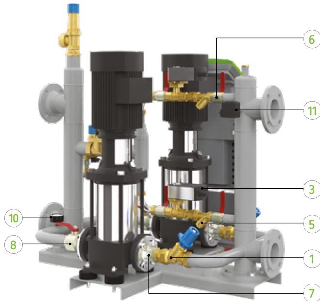
Variomat Giga Hydraulikmodul – Rückansicht
