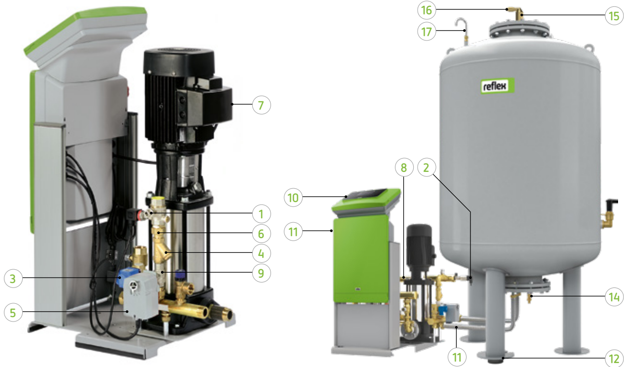
Variomat Steuereinheit – Rückansicht
