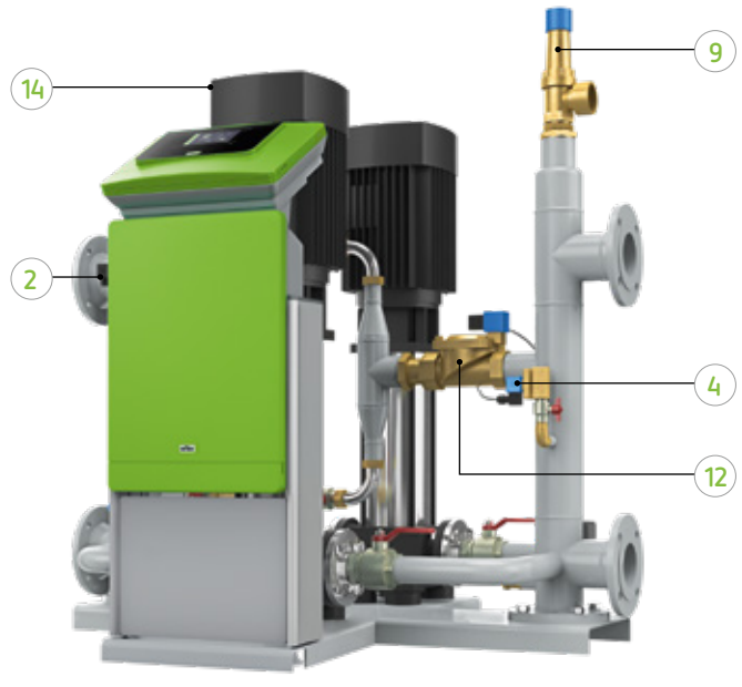
Variomat Giga Steuerung und Hydraulikmodul
