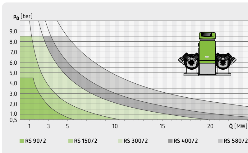
Reflexomat se dvěma kompresory
