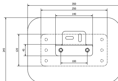
PV-Halter klein
