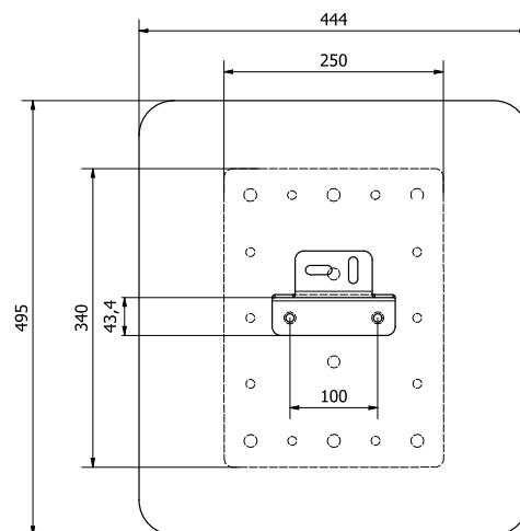
PV-Halter groß
