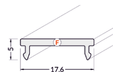
Transparent/opal täcklock
