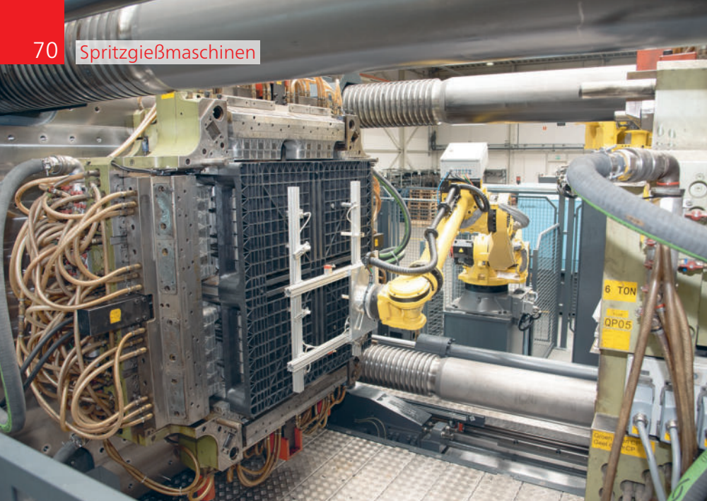
Bei der Palettenproduktion aus Post-Consumer-Rezyklat wird während des Zyklus kontinuierlich plastifiziert und über ein Kolbenaggregat der Kavität zugeführt. Die Entnahme sowie die Ablage der Palette erfolgen automatisiert.
